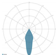
ÓPTICAS: 4-ROSOSIMÉTRICA 30°
