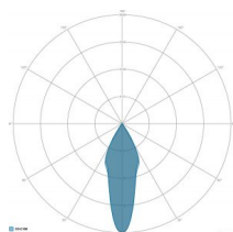
ÓPTICAS: 4-ROSOSIMÉTRICA 30°
