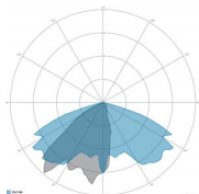
ÓPTICAS: 7-ASIMÉTRICA VIAL
