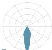
ÓPTICAS: 4-ROSIMÉTRICA 30°
