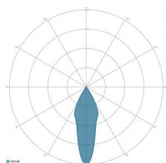
ÓPTICAS: 4-ROTOSIMÉTRICA 30°
