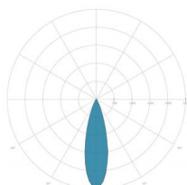
ÓPTICAS: 5-RODOSIMÉTRICA 20°
