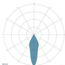
ÓPTICAS: 4-ROTSIMÉTRICA 30°
