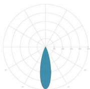
ÓPTICAS: 5-ROTSIMÉTRICA 20°
