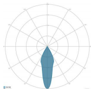
ÓPTICAS: 4-RODOSIMÉTRICA 30°
