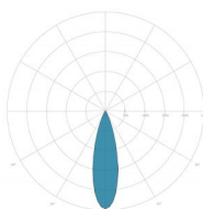
OTTICA: 5-ROTOSIMMETRICA 20°
