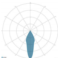
OTTICA: 4-ROTOSIMMETRICA 30°
