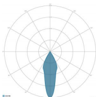
OTTICA: 4-ROTSIMMETRICA 30°
