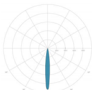
OTTICA: 6-ROTOSIMMETRICA 10°
