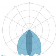
OTTICA: 3-SIMMETRICA SPORT STRETTA
