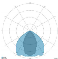
OTTICA: 2-SIMMETRICA LARGA
