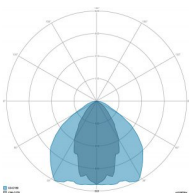
OTTICA: 2-SIMMETRICA LARGA
