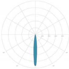
OTTICA: 6-ROTOSIMMETRICA 10°
