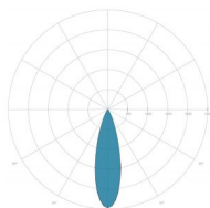
OTTICA: 5-ROTOSIMMETRICA 20°
