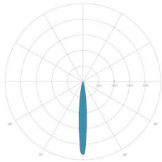
OTTICA: 6-ROTSIMMETRICA 10°
