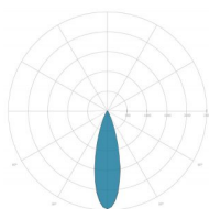
OTTICA: 5-ROTOSIMMETRICA 20°
