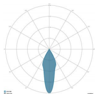
OTTICA: 4-ROSIMMETRICA 30°
