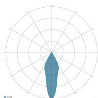
OTTICA: 4-ROSI-METRICA 30°
