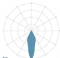
OTTICA: 4-ROTOSIMMETRICA 30°
