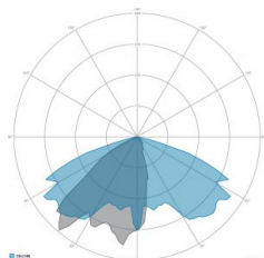
OTTICA: 7-ASIMMETRICA STRADALE
